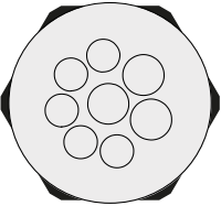
KEL-DPZ 50|8 CR gy
